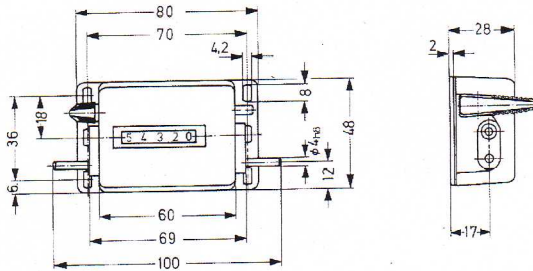
Dimensions M300/M310
